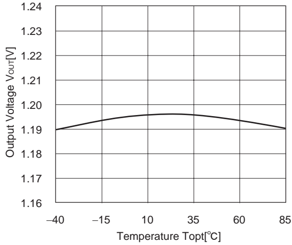
R1180x121x ( V_{IN}=2.2V )
