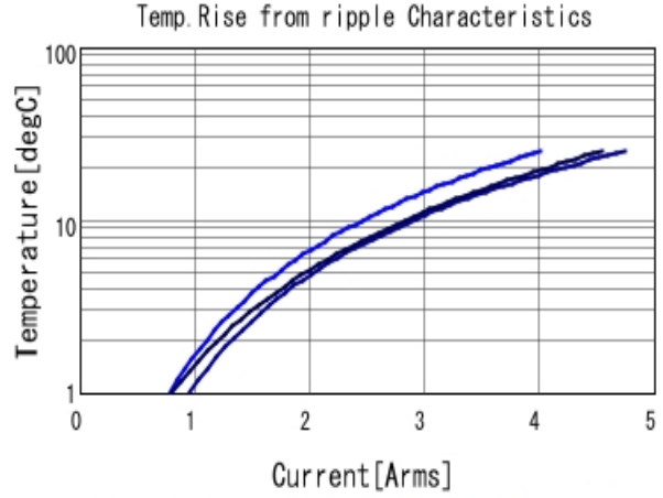
KCM55TR72A106MH01 Temp. rise ■ 50kHz ■ 100kHz ■ 300kHz
