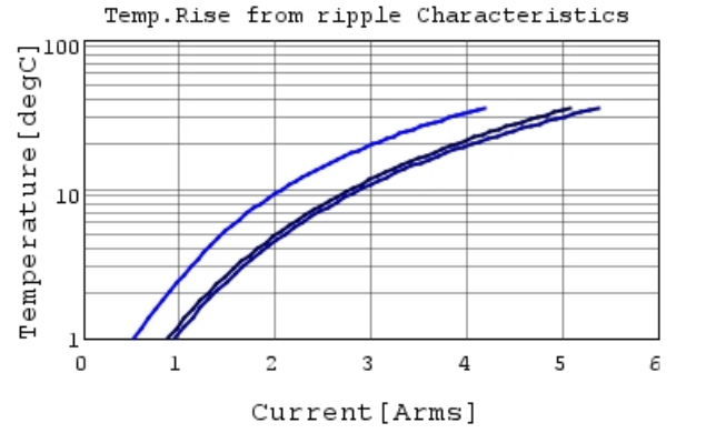
GRM31CR61H106KA12 Temp.rise 100kHz
