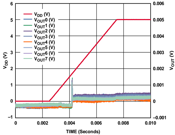
Figure 41. POR to 0 V Output
