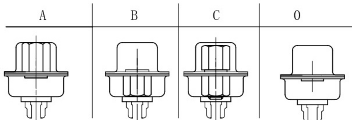
铆钉型式
