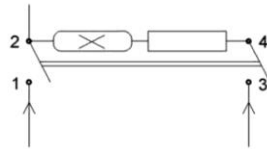
Электрическая схема коммутации
