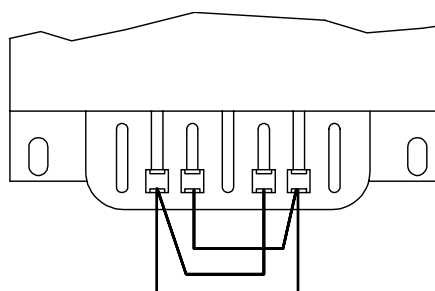
Fonctionnement 115 V
