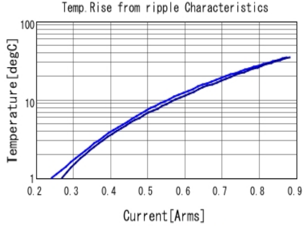
GJM1555C1H1R2BB01 Temp. rise ■ 2GHz ■ 3GHz
