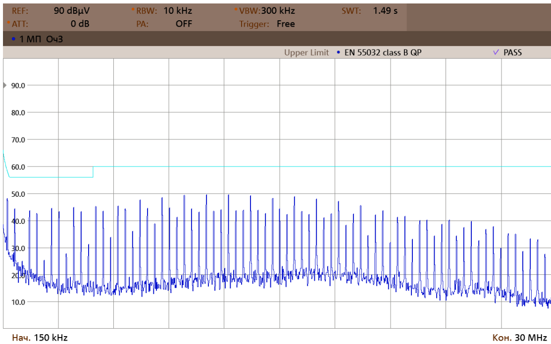
Рис. 37. Спектрограмма соответствия EN55032 Class B (0,15–30 MHz).
