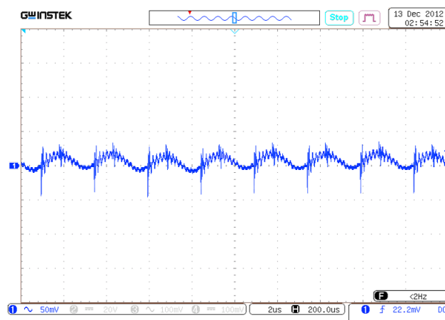
Рис. 29. Осциллограмма пульсаций U_{\text{ВЫХ.НОМ}} .
