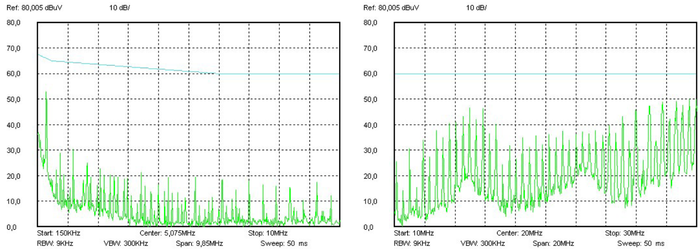
Рис. 11 (а). Спектрограммы 0,01–10 MHz.
