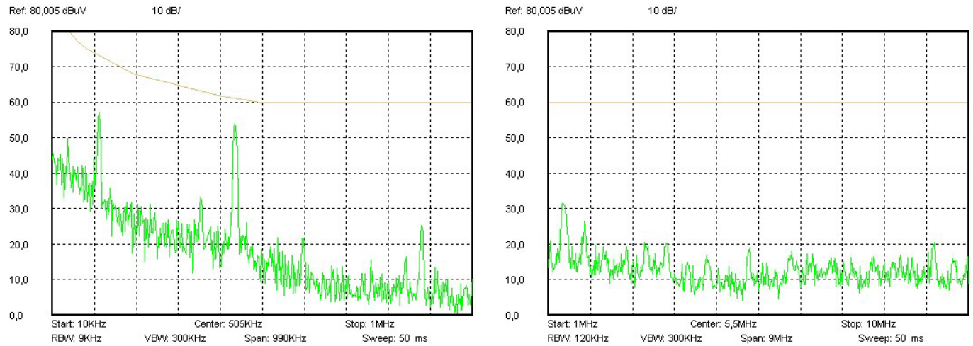
Рис. 12 (а). Спектрограммы 0,01–10 MHz.
