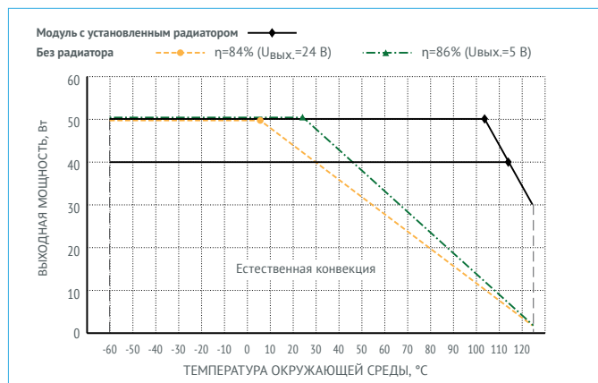
Рис. 8. Тепловая кривая VDR40 и VDR50.
