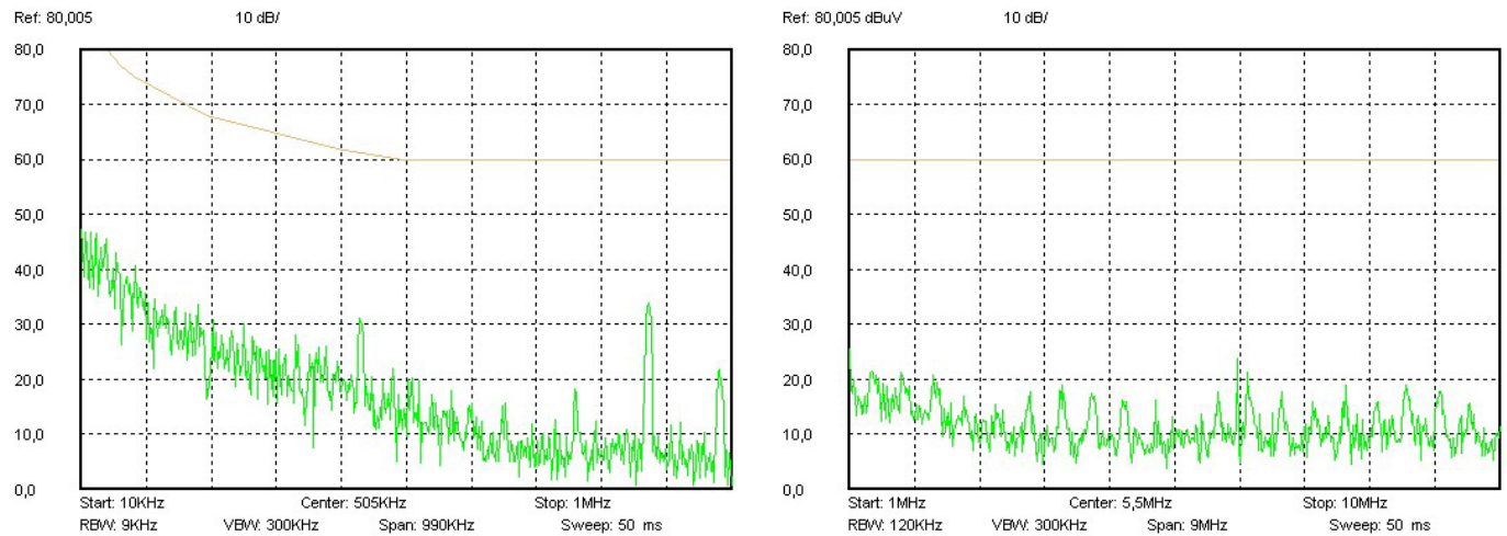
Рис. 12 (б). Спектрограммы 0,01–10 MHz.
