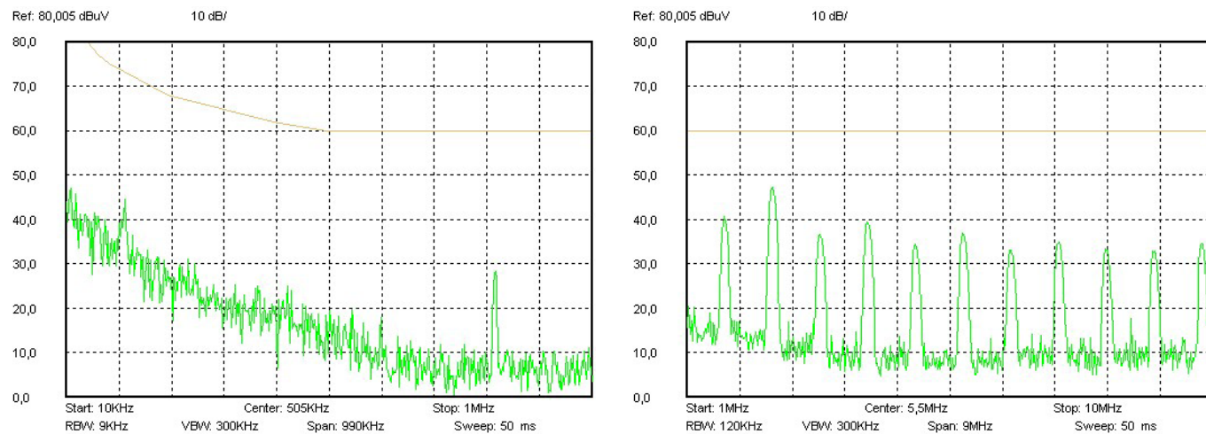
Рис. 14 (а). Спектрограммы 0,01–10 MHz.
