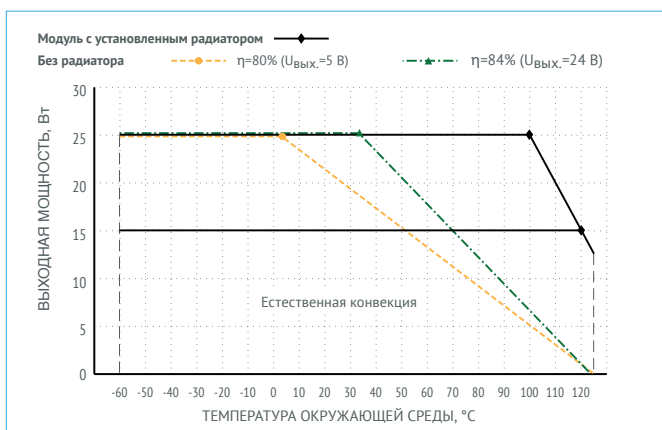
Рис. 10. Тепловая кривая VDR15 и VDR25.
