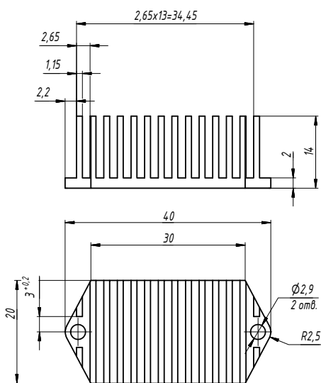
Рис. 17 (а). ТУЛВ. 752694.001.
