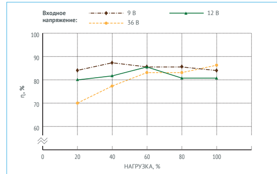
Рис. 9 (б). КПД VDR25B24.
