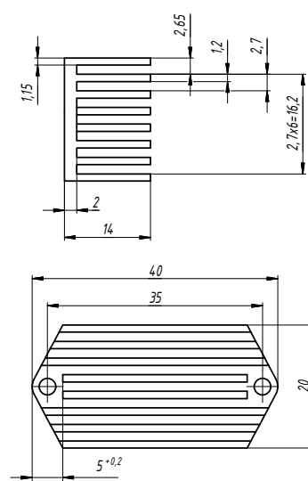
Рис. 17 (б). ТУЛВ. 752694.002.
