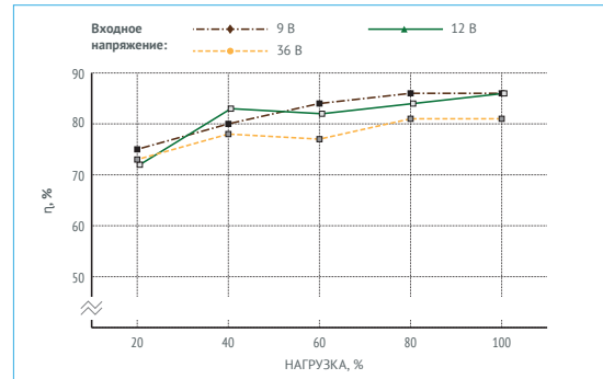
Рис. 7 (е). КПД VDR15B24.
