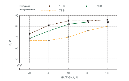
Рис. 8 (б). КПД VDR15BW05.
