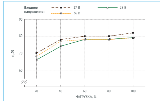
Рис. 6 (б). КПД VDR10V05.
