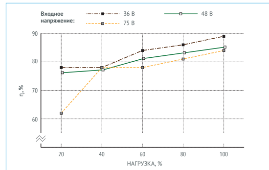
Рис. 7 (б). КПД VDR10D15.
