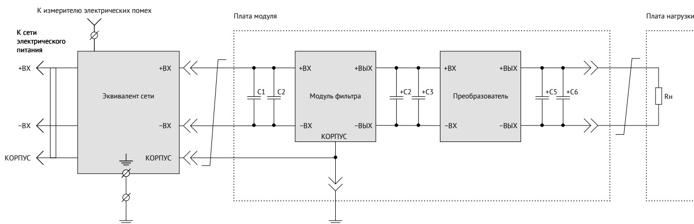
Рис. 5. Схема включения VDRI6, VDRI10.
