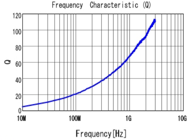
■ LQW15AN8N7J00 Q
