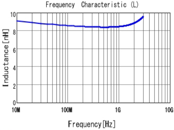
■ LQW15AN8N7J00 L
