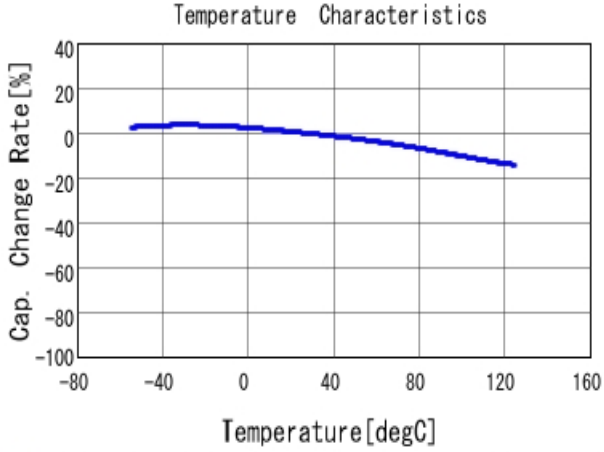
■ GRM32ER71A226ME20 C-Temp. capchange, DCO. 0V, ACO. 5V rm
