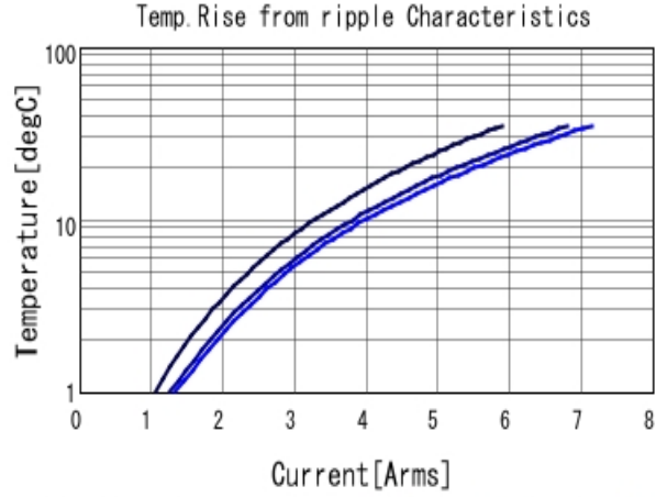
GRM32ER71A226ME20 Temp. rise ■ 100kHz ■ 500kHz ■ 1MHz
