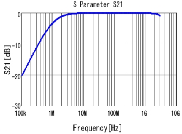
■ GA342QR7GD152KW01 S21 DCOV, 25degC
