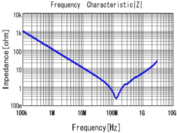
■ GA342QR7GD152KW01 |Z| DC0V, 25degC
