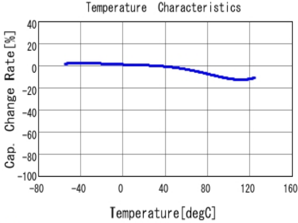
■ GA342QR7GD152KW01 C-Temp. capchange, DCOV, AC1Vrms
