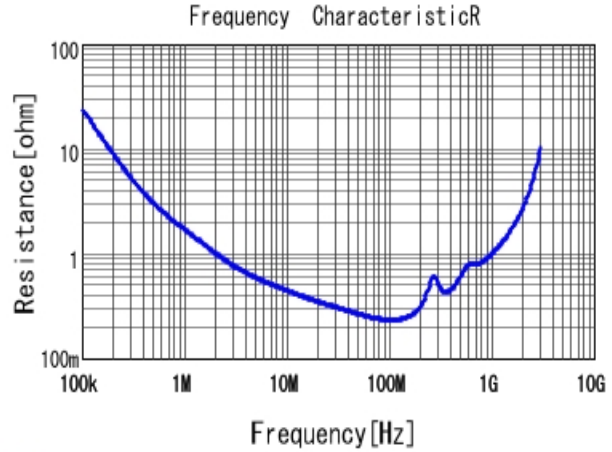
■ GA342QR7GD152KW01 R DC0V, 25degC
