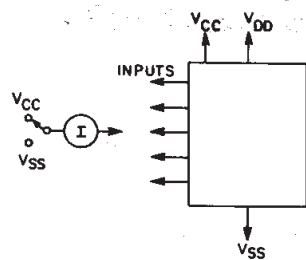
Fig. 7 - Input current.
