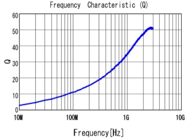
■ LQG15HN4N3S02 Q
