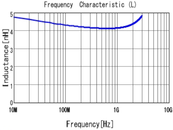
■ LQG15HN4N3S02 L
