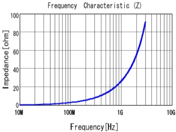
■ LQG15HN4N3S02 |Z|
