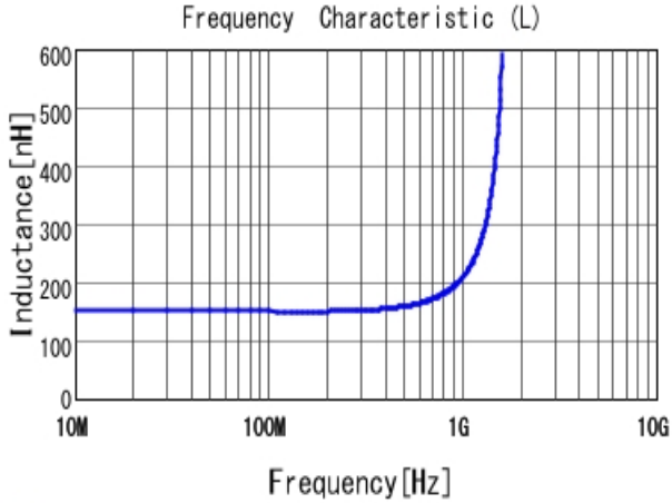
■ LQW18ANR15G00 L
