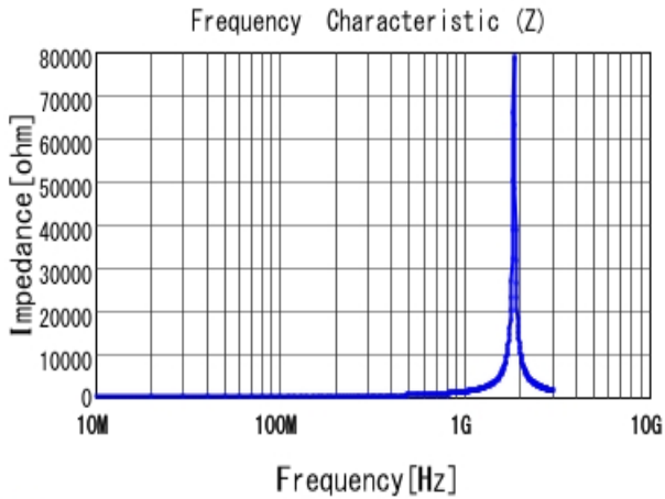
■ LQW18ANR15G00 |Z|
