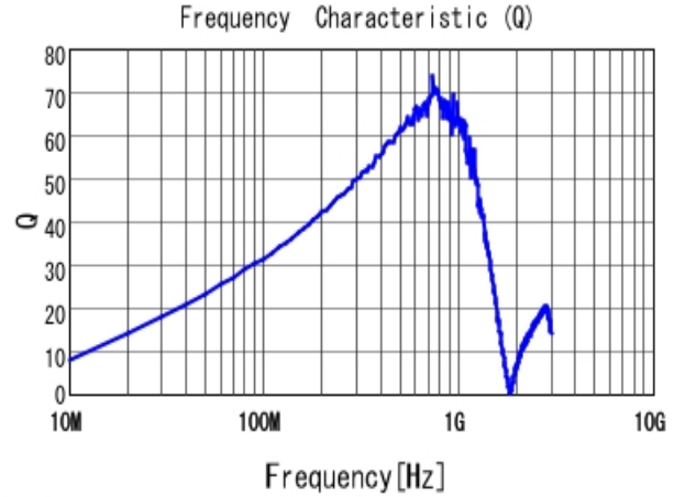
■ LQW18ANR15G00 Q
