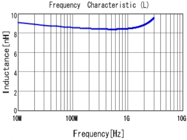
■ LQW15AN8N7G00 L
