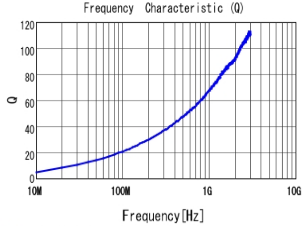
■ LQW15AN8N7G00 Q
