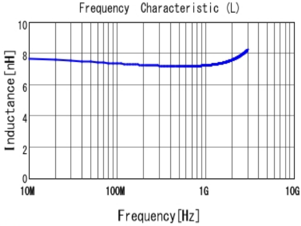
■ LQW15AN7N5G00 L
