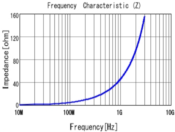
■ LQW15AN7N5G00 |Z|
