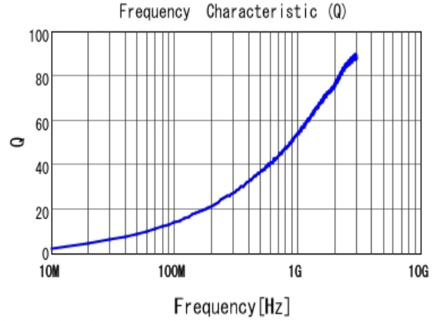
■ LQW15AN7N5G00 Q
