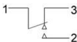
Электрическая схема коммутации
