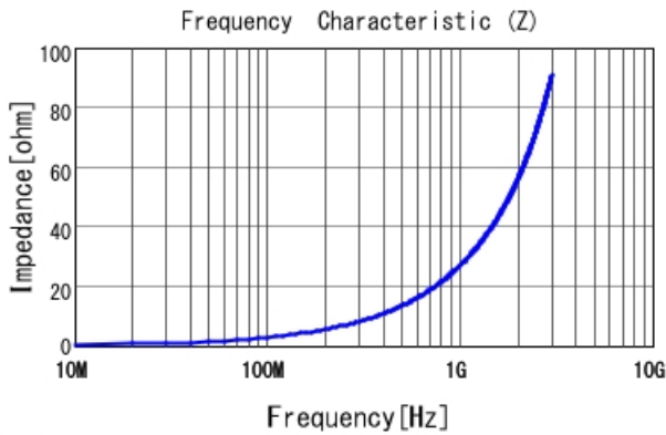
■ LQP03TN4N3H02 |Z|
