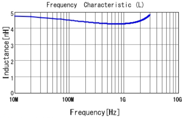
■ LQP03TN4N3H02 L
