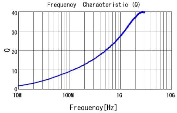
■ LQP03TN4N3H02 Q
