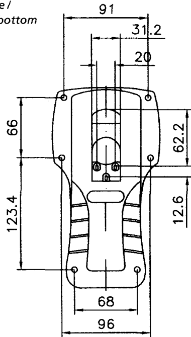
Unterschale / enclosure bottom
