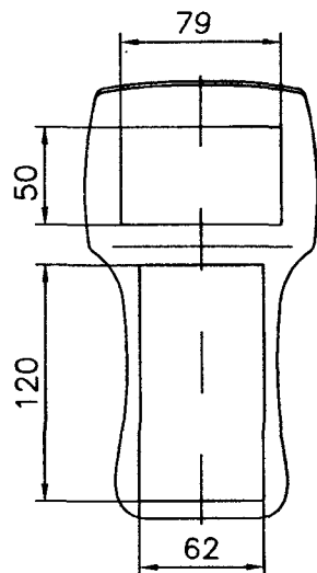
Oberschale / enclosure top
