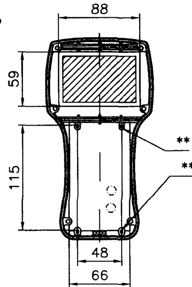
Oberschale / enclosure top
