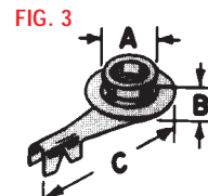
Stud w/Crimp Lugon
