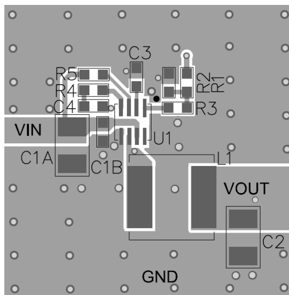
Top Layer
