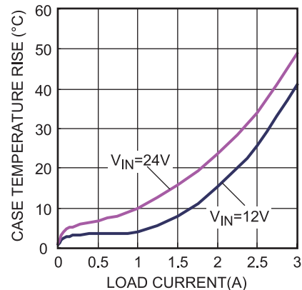
Thermal Rise
