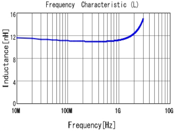
■ LQW18AN11NG00 L
