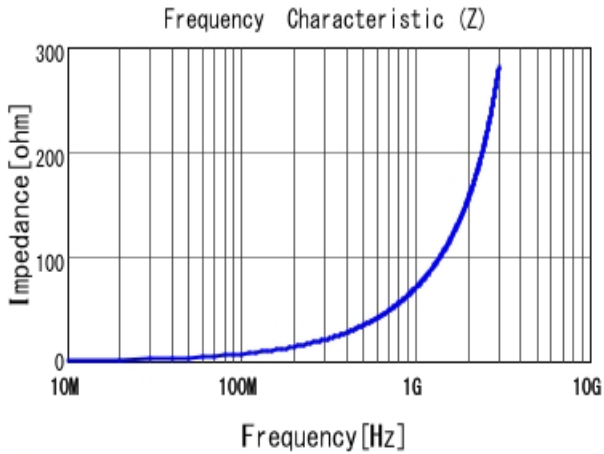
■ LQW18AN11NG00 |Z|
