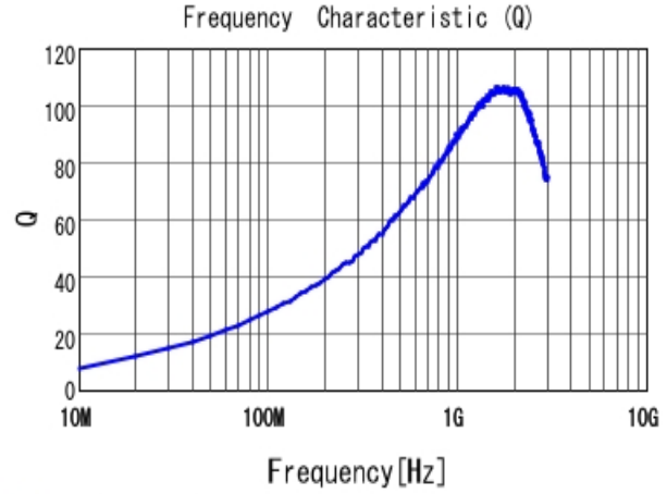
■ LQW18AN11NG00 Q
