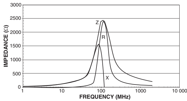
ILBB-0805 2200 Ω
