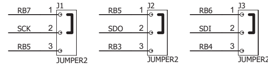
AVR 28pin
