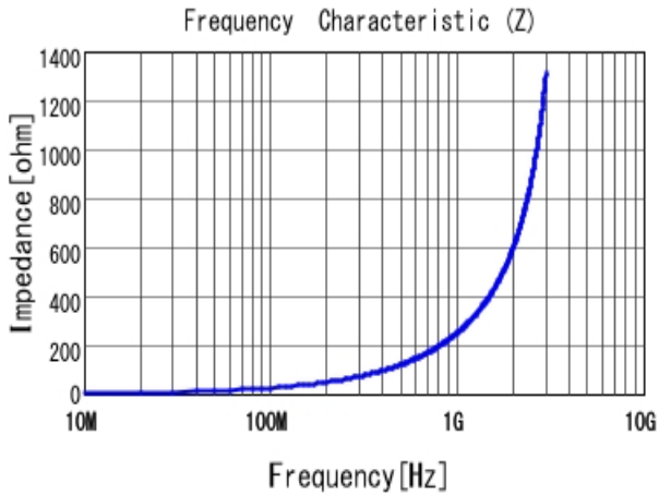
■ LQW15AN39NG00 |Z|
