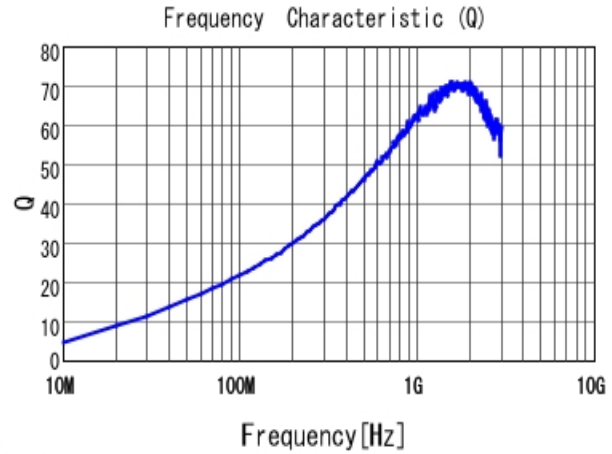
■ LQW15AN39NG00 Q
