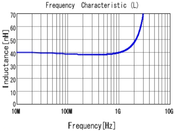
■ LQW15AN39NG00 L
