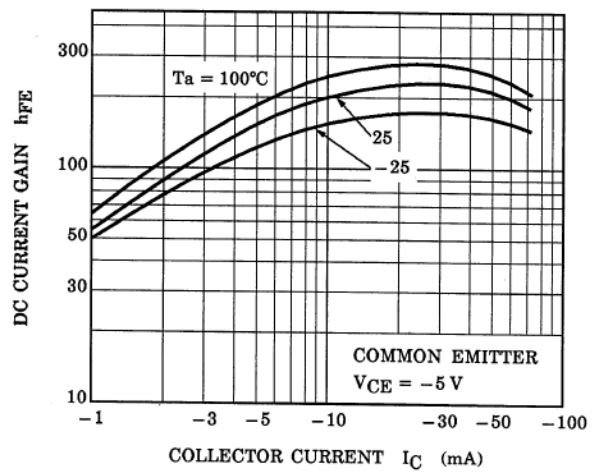
Fig. 10.16 RN2404 h_{FE}-I_C
