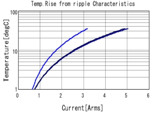
GRM31MR71A225KA01 Temp. rise ■ 100kHz ■ 500kHz ■ 1MHz
