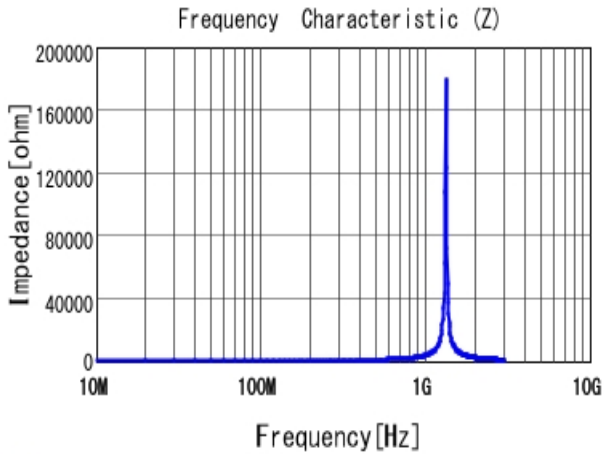
■ LQW18ANR27J00 |Z|
