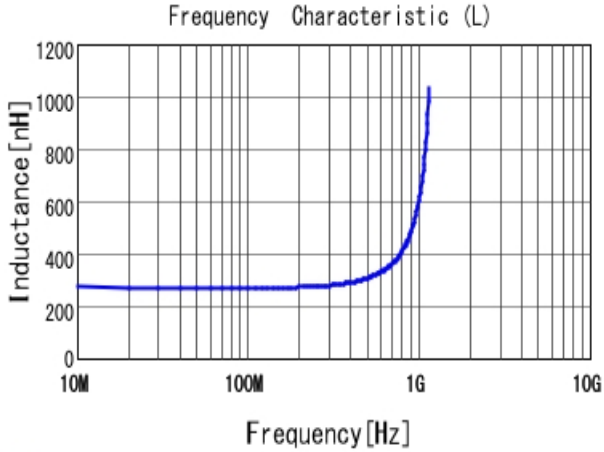
■ LQW18ANR27J00 L
