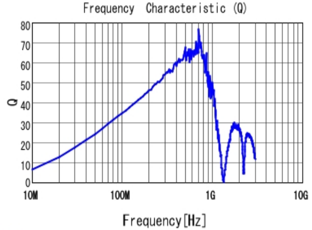
■ LQW18ANR27J00 Q
