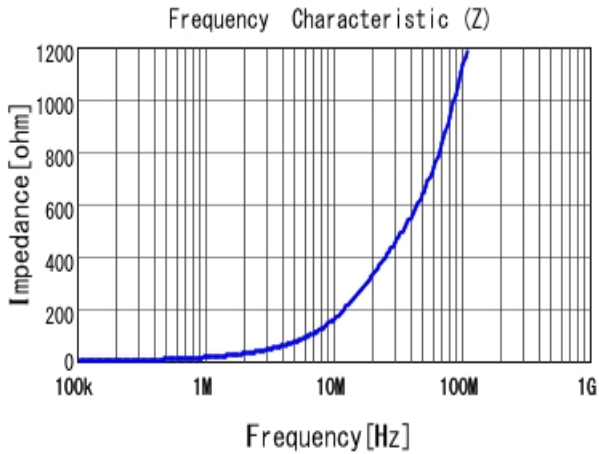
■ LQM18PN2R2MFR |Z|
