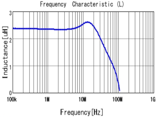
■ LQM18PN2R2MFR L
