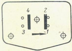
Рис. 23. Схема коммутации выключателя ВБТ-1 и переключателя ТВ1-1
