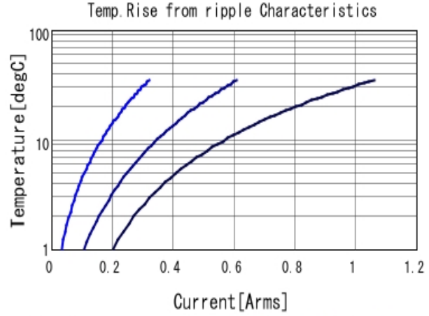
GRM43DR73A473KW01 Temp. rise ■ 30kHz ■ 100kHz ■ 300kHz
