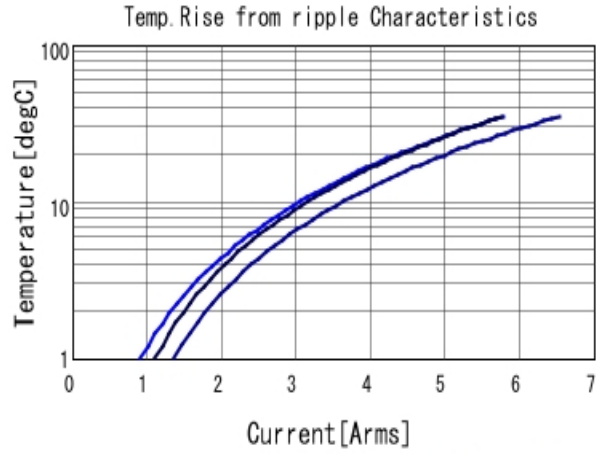
GRM32EC81C476ME15 Temp. rise ■ 60kHz ■ 300kHz ■ 600kHz
