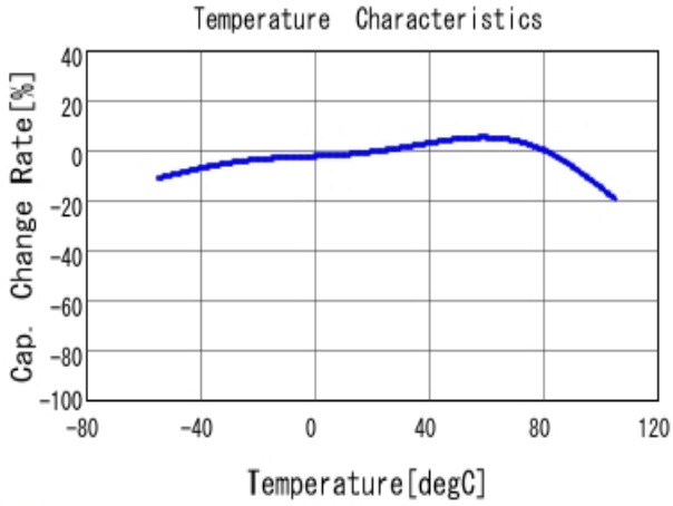
■ GRM32EC81C476ME15 C-Temp. capchange, DCO. 0V, ACO. 5V rm
