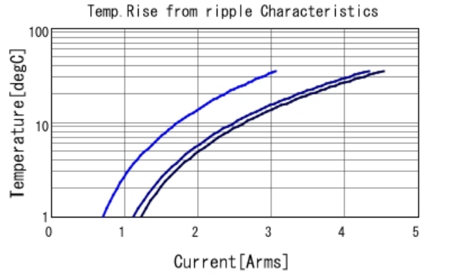
GRM155R60G475ME87 Temp. rise — 100kHz — 500
