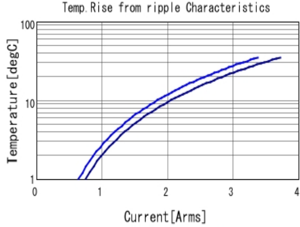
GRM155C81C225KE11 Temp. rise ■ 500kHz ■ 1MHz
