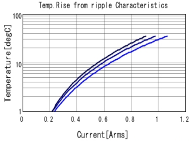
GRM1555C1E180JA01 Temp. rise ■ 500MHz ■ 700MHz ■ 1GHz
