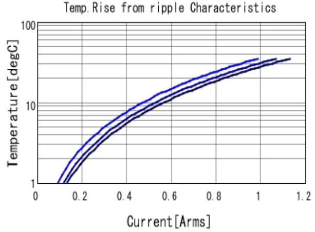
GRM033C81E104KE14 Temp. rise ■ 400kHz ■ 800kHz ■ 1MHz
