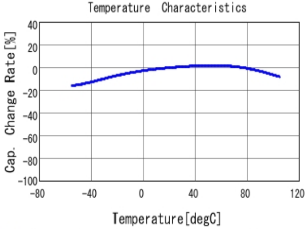
■ GRM033C81E104KE14 C-Temp. capchange, DCO. 0V, ACO. 2V rm
