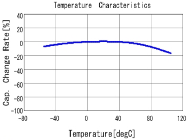
■ GRM033C80J223KE01 C-Temp. capchange, DCO. 0V, ACO. 5Vrm
