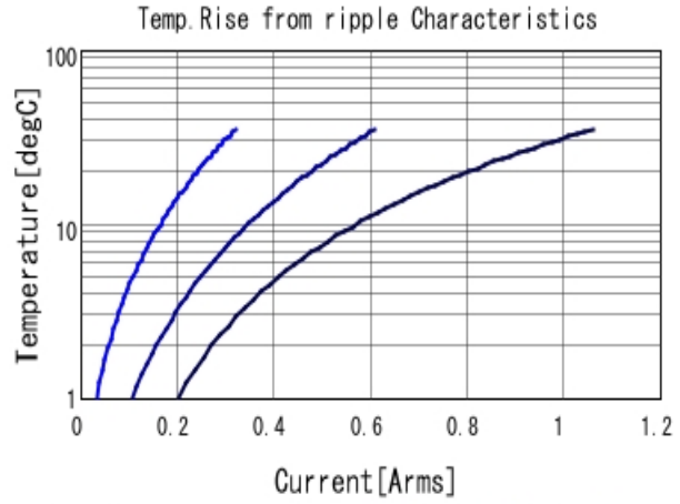
GCJ43DR72J473KXJ1 Temp. rise 30kHz 100kHz 300kHz
