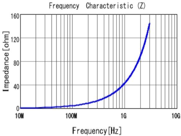
■ LQW15AN6N8J00 |Z|
