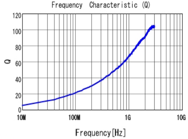
■ LQW15AN6N8J00 Q
