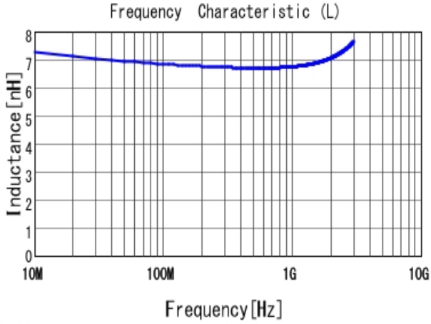
■ LQW15AN6N8J00 L
