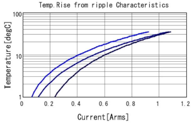
GRM033C71A104KE14 Temp. rise ■ 400kHz ■ 800kHz ■ 1MHz
