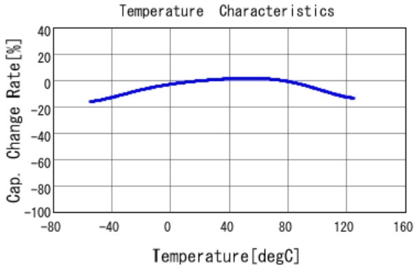
■ GRM033C71A104KE14 C-Temp. capchange, DCO. 0V, ACO. 2Vrm
