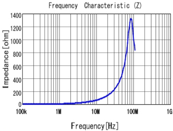
■ LQM31PN1R0M00 |Z|
