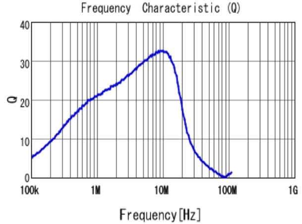
■ LQM31PN1R0M00 Q
