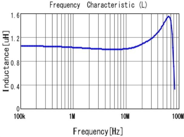
■ LQM31PN1R0M00 L
