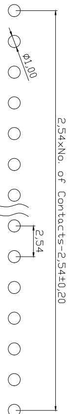
P.C.B. LAYOUT
