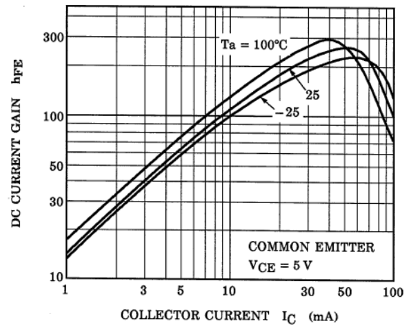
Fig. 10.14 RN1102 h_{FE}-I_C
