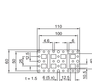
TS 4532.000 Verschraubbar, klein
