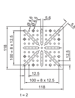
TS 8612.410 Verschraubbar, groß
