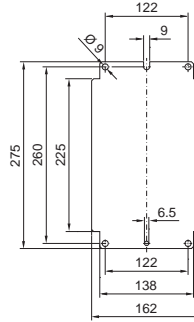
Montageplatten AE 1001.X00, AE 1002.X00
