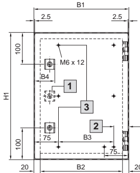
AE 1001.X00 – AE 1016.X00
