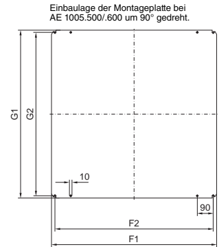
Montageplatten AE 1018.X00
