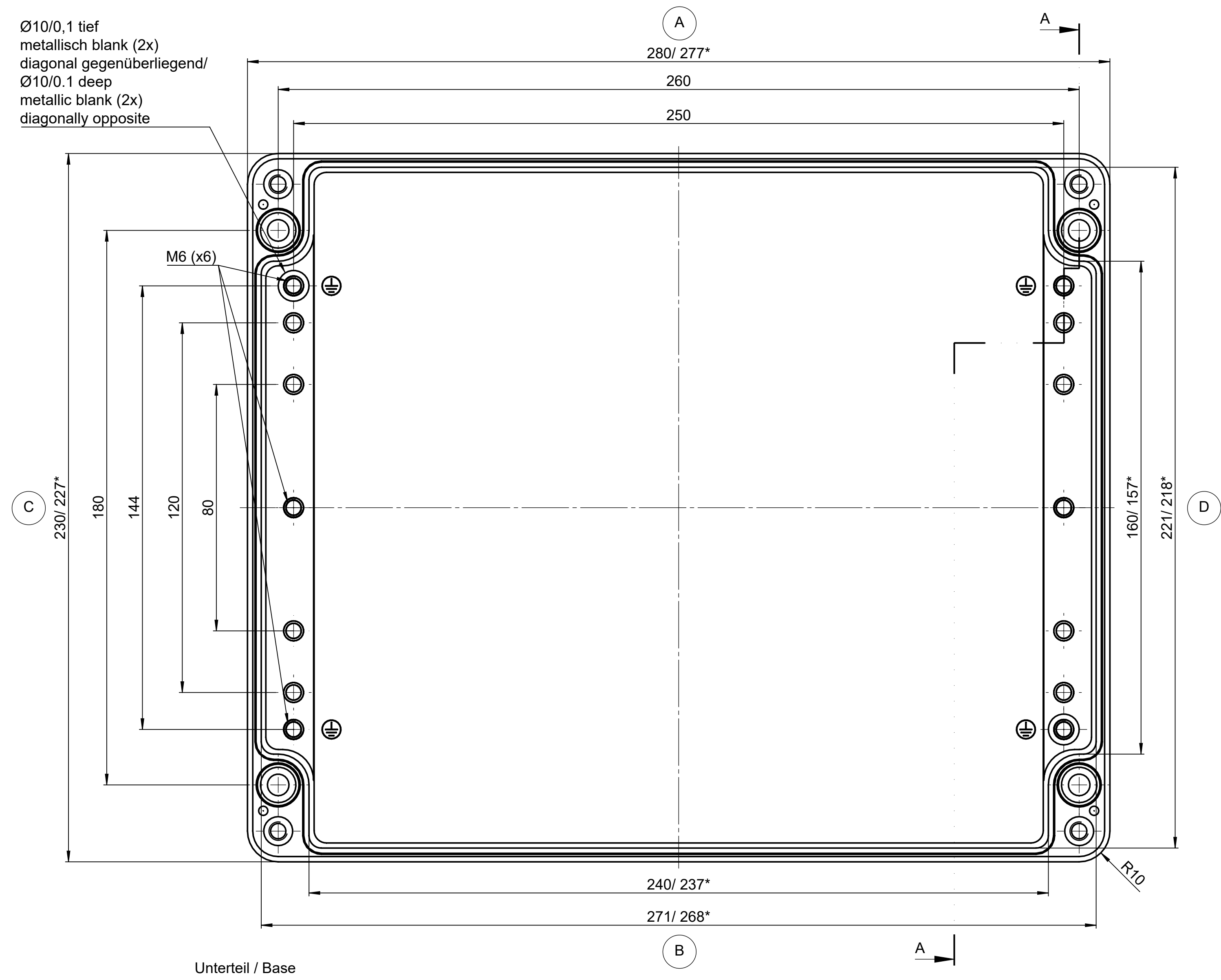
Unterteil / Base
